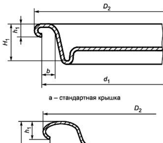
Рисунок 2 - Параметры и размеры крышек
